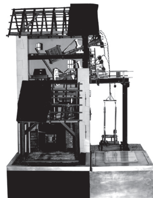
Model Potterovho atmosférického stroja; zbierkový fond Pohronského múzea.
